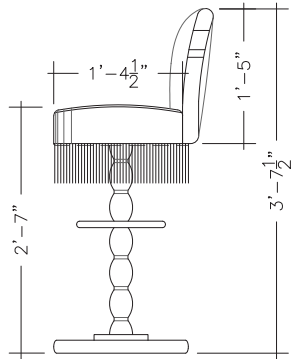
BAR STOOL - SIDE
