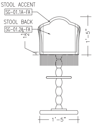
BAR STOOL - BACK
